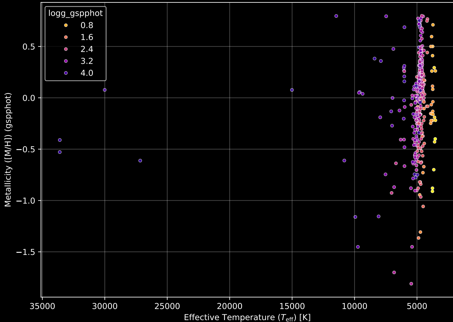
APOGEE DR17 Field: [000-04] Stellar Population Parameters (n= 405)
